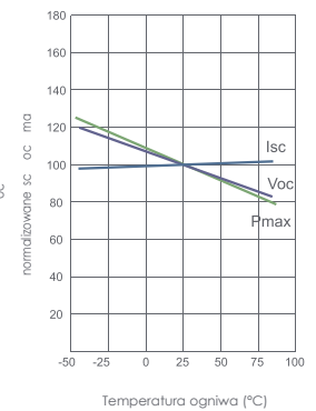
Zależność temperatury I sc , V oc , P max
